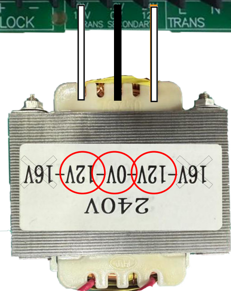
12v 0v 12v(5A)
